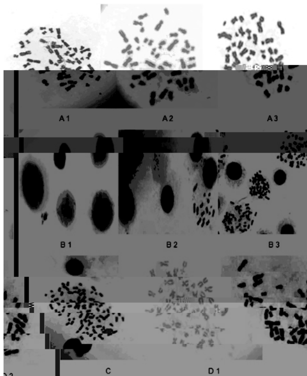
注:A1~A3 表示优化后的染色体核型;B1~B2 表示低渗时间小于或等于 15 min;B3 表示低渗时间等于 20 min;C 表示固定时间小于或等于 20 min;D1 表示染色时间小于或等于 15 min;D2 表示染色时间大于或等于 25 min。
